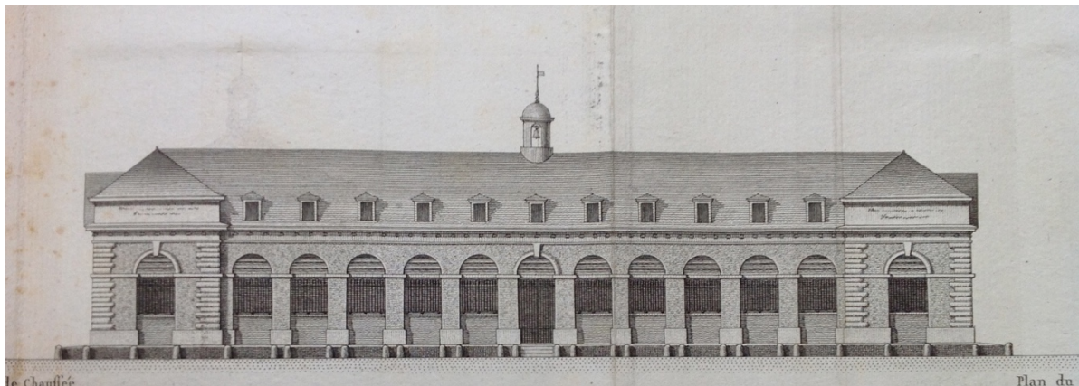
Élévation de la halle au bled de la ville de Corbeil
